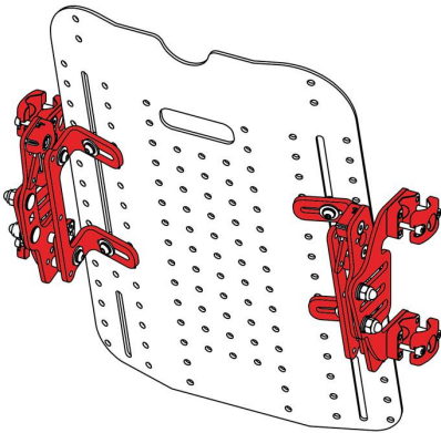
Soporte de 2 puntos «Dual Mount»
